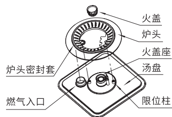
双灶炉头、火盖安装示意图
