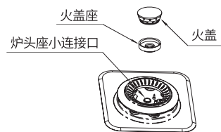
单灶火盖安装示意图
