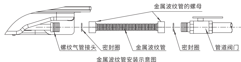
金属波纹管安装示意图
