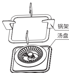
锅架安装示意图
